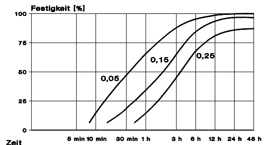
Aushärtung in Abhängig. v. Spalt Test in Anlehnung an DIN 54 454
