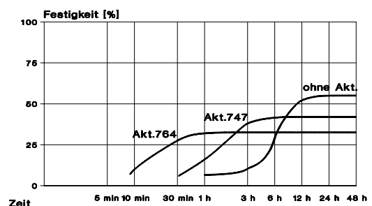
Aushärtung in Abhängig. v. Aktivator Test in Anlehnung an DIN 54 454
