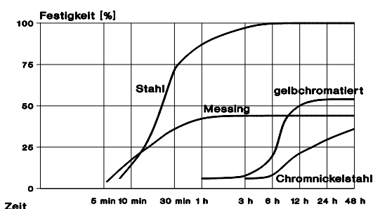
Aushärtung in Abhängig. v. Material Test in Anlehnung an DIN 54 454
