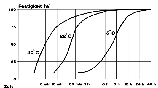
Aushärtung in Abhängig. v.d Temperatur Test in Anlehnung an DIN 54 454
