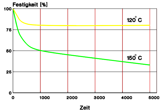
Wärmealterung Test in Anlehnung an DIN 54 452
