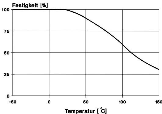
Festigkeit in Abhängigk. v.d. Temperatur Test in Anlehnung an DIN 53 286
